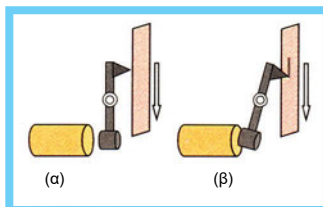
Σχήμα 2.4.3 Τηλεγραφικό πλήκτρο.
