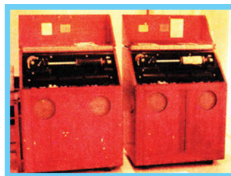
Σχήμα 2.11.1 Το αναλογικό τηλεομοίτυπο (φαξ) του 1935. Από το Μουσείο Τηλεπικοινωνιών του ΟΤΕ.
