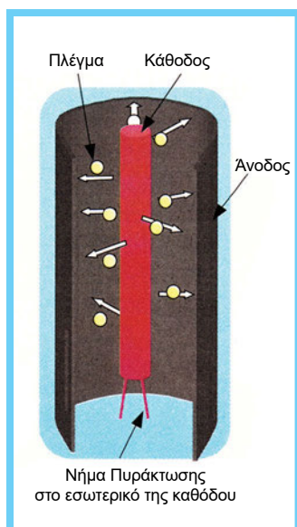
Σχήμα 2.9.3 Η δίοδος λυχνίας στην οποία φαίνεται με βέλη η κίνηση των ηλεκτρονίων από την πυρακτωμένη κάθοδο προς την άνοδο.
