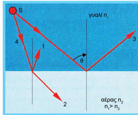
Σχήμα 3.4.1 Οι ακτίνες της πηγής S κατευθύνονται από μέσο με μεγάλο δείκτη διάθλασης (δ.δ.), σε μέσο με μικρό δ.δ.
