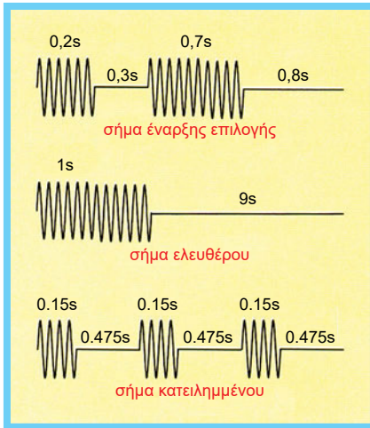
Σχήμα 7.3.1 Οι διάρκειες των (ηχο)σημάτων.
