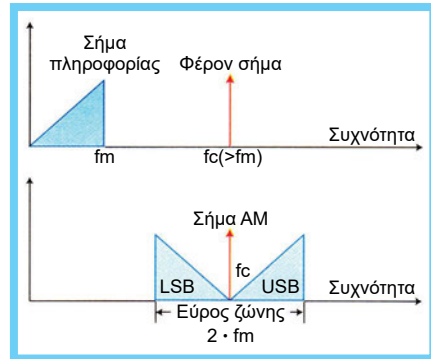
Σχήμα 5.10.4 Φασματικό περιεχόμενο ενός AM σήματος.
